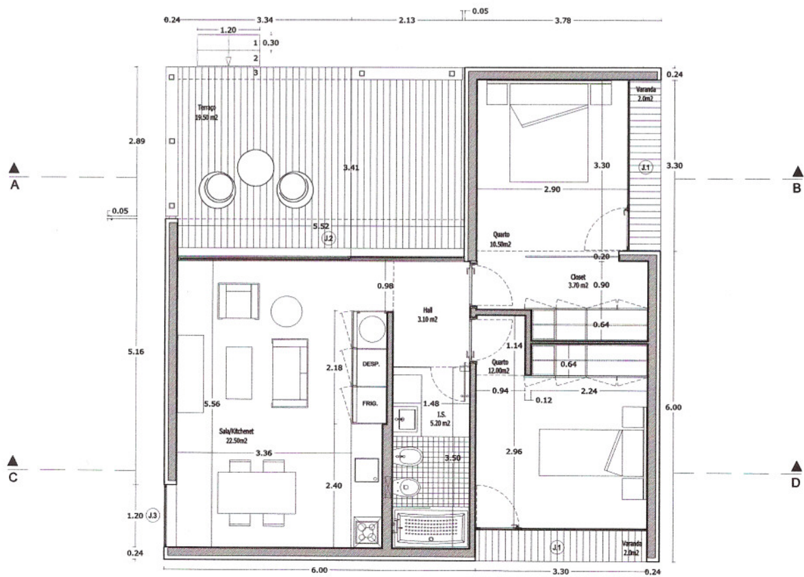
PLANTA de PISO
